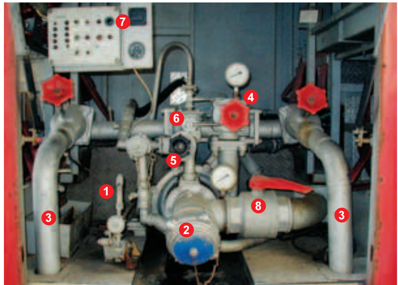
1 - ручка "газа" (напор); 2 - центральный патрубок (здесь заливается вода) 3 - сюда цепляют рукава; 4 - центральный кран 5 - вентиль бака с пеной; 6 - ручка смесителя с пеной; 7 - датчики; 8 - кран центрального патрубка
